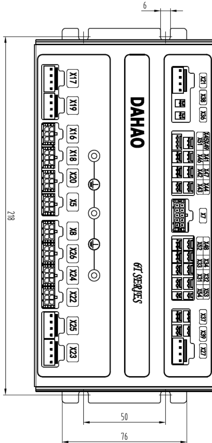
Schema dell'interfaccia del cablaggio posteriore del control box
